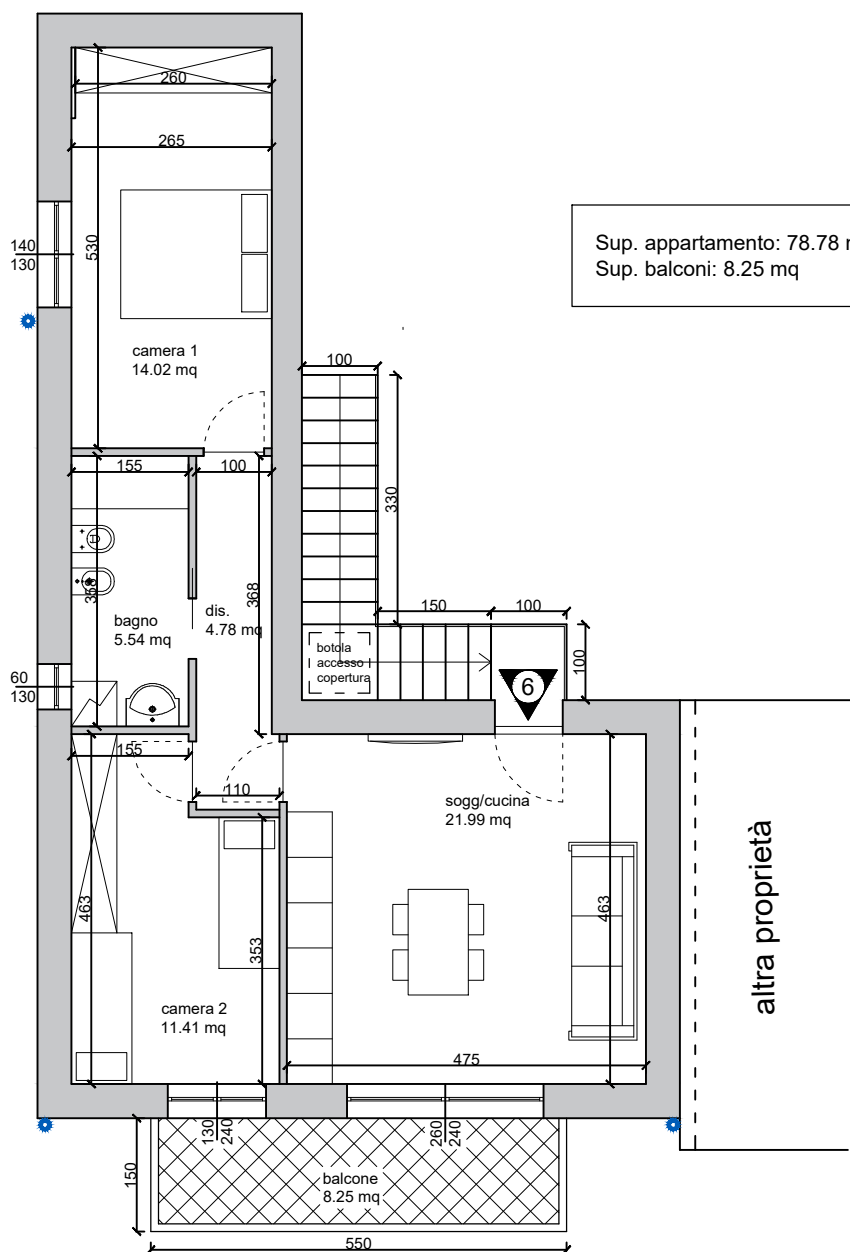
PIANO SECONDO_appartamento 6
